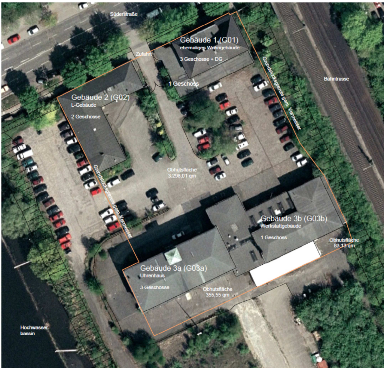
Lageplan 1:500 Quelle Luftbild: Google maps; Flächenangaben Obhutsflächen (Fläche um Gebäude) gem. Vermesser
